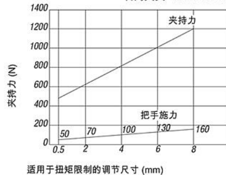
转角夹具 04366-...4540
