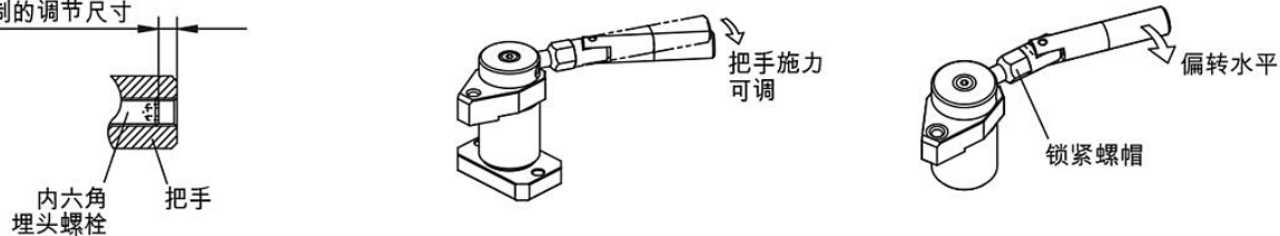
适用于扭矩限制的调节尺寸
