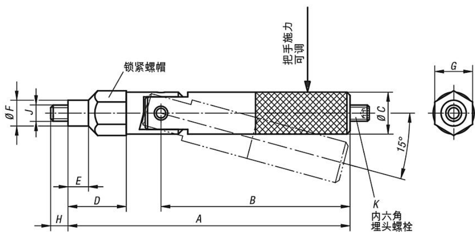
适用于扭矩限制的调节尺寸
