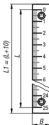
带孔 垂直安装位置
