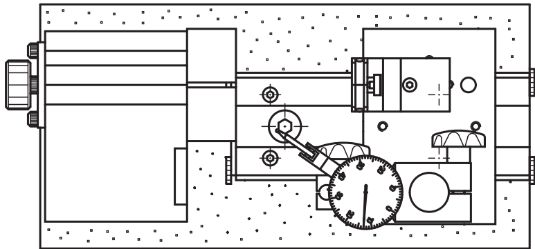
以棱柱作为长部件托架支撑的示例
