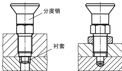
定位 带定位衬套
