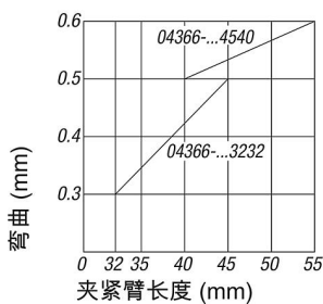
夹紧时 弯曲的夹紧臂长度 C
