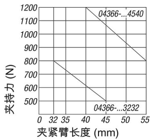
相对夹持力的夹紧臂长度 C
