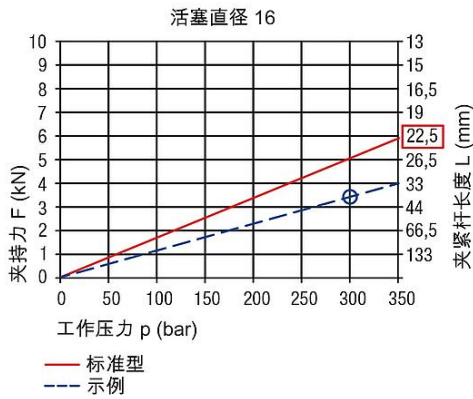
夹紧力示意图
